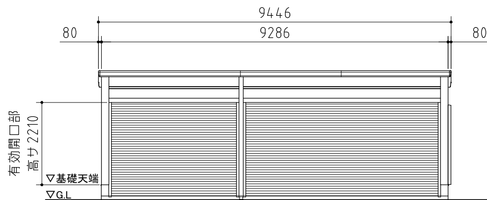
正面図
